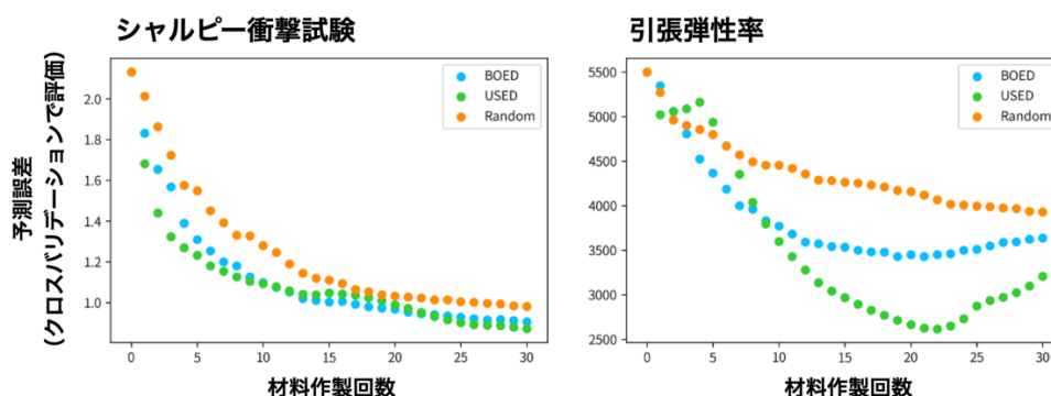
図3 シャルピー衝撃試験（左図）および引張弾性率（右図）に対する予測誤差の材料作製回数依存性。本研究で考案したベイズ最適化に基づく手法（BOED）および不確実性サンプリングに基づく手法（USED）、無作為に実験を行う手法（Random）を比較しています。Randomに比べて、BOEDおよびUSEDを用いることで少ない材料作製回数でも予測誤差が小さくなっていることがわかります。つまり、本研究で開発した新AI技術を利用することで、少ない作製回数で材料予測の精度向上を達成できました。
